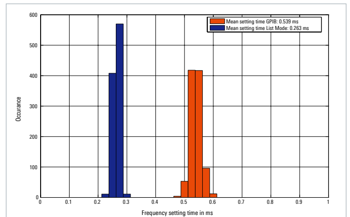
在使用GPIB控制和列表模式下，超过1000次频率设置时间测量的柱状图
