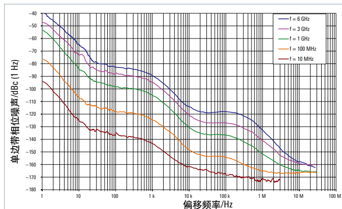
测量内部基准振荡器单边带相位噪声 (标准仪器配置)
