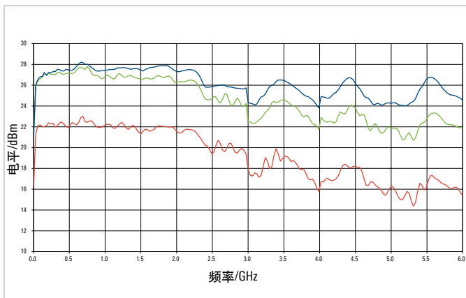
最大可用功率、衰减器模式NORMAL（下部迹线）或HIGH POWER（中间迹线），以及不使用衰减器时（上部迹线）
