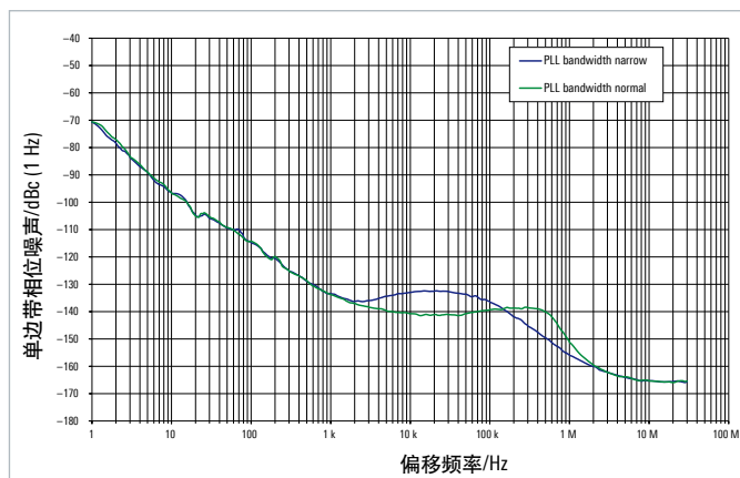
锁相环路带宽在正常和窄带模式下 ( f \leq 3 GHz)，测得单边带相位噪声 (使用R&S®SMA-B22增强型相位噪声性能和FM/φM调制器选件)
